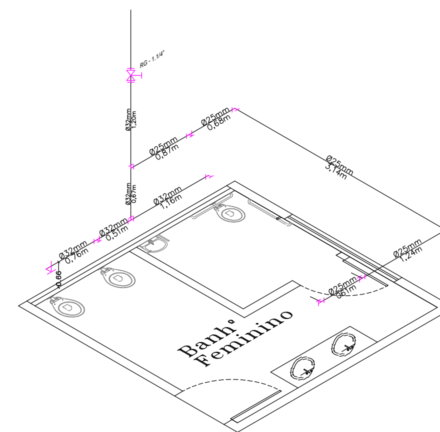
ISOMÉTRICO: BACIAS SANITÁRIAS E LAVATORIOS escala: 1:50 Tubo \varnothing 25mm=(0,87m+0,68m+3,14m+1,24m+0,61m)=6,54m. Tubo \varnothing 32mm=(1,20m+0,67m+1,16m+0,51m+0,75m)=4,30m. Reg. Gaveta 1"=1,0 uni.
