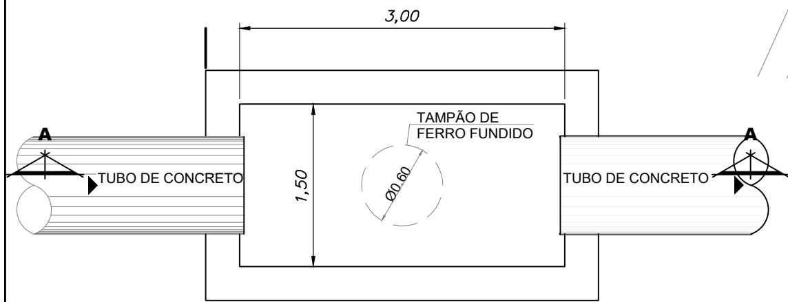
PLANTA BAIXA BASE POÇO DE VISITA Sem Escala
