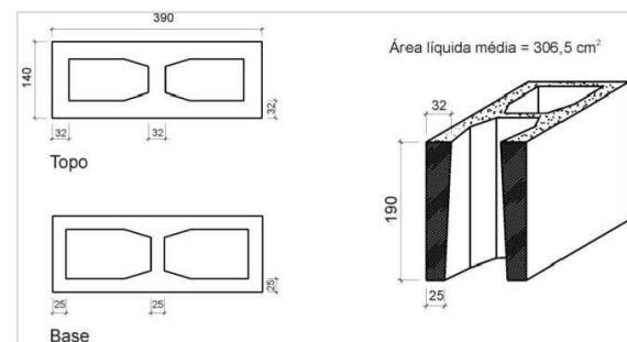
DETALHE BLOCO DE CONCRETO Sem Escala
