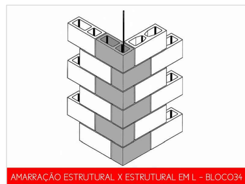
DETALHE AMARRAÇÃO Sem Escala
