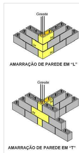
DETALHE GRAUTE Sem Escala
