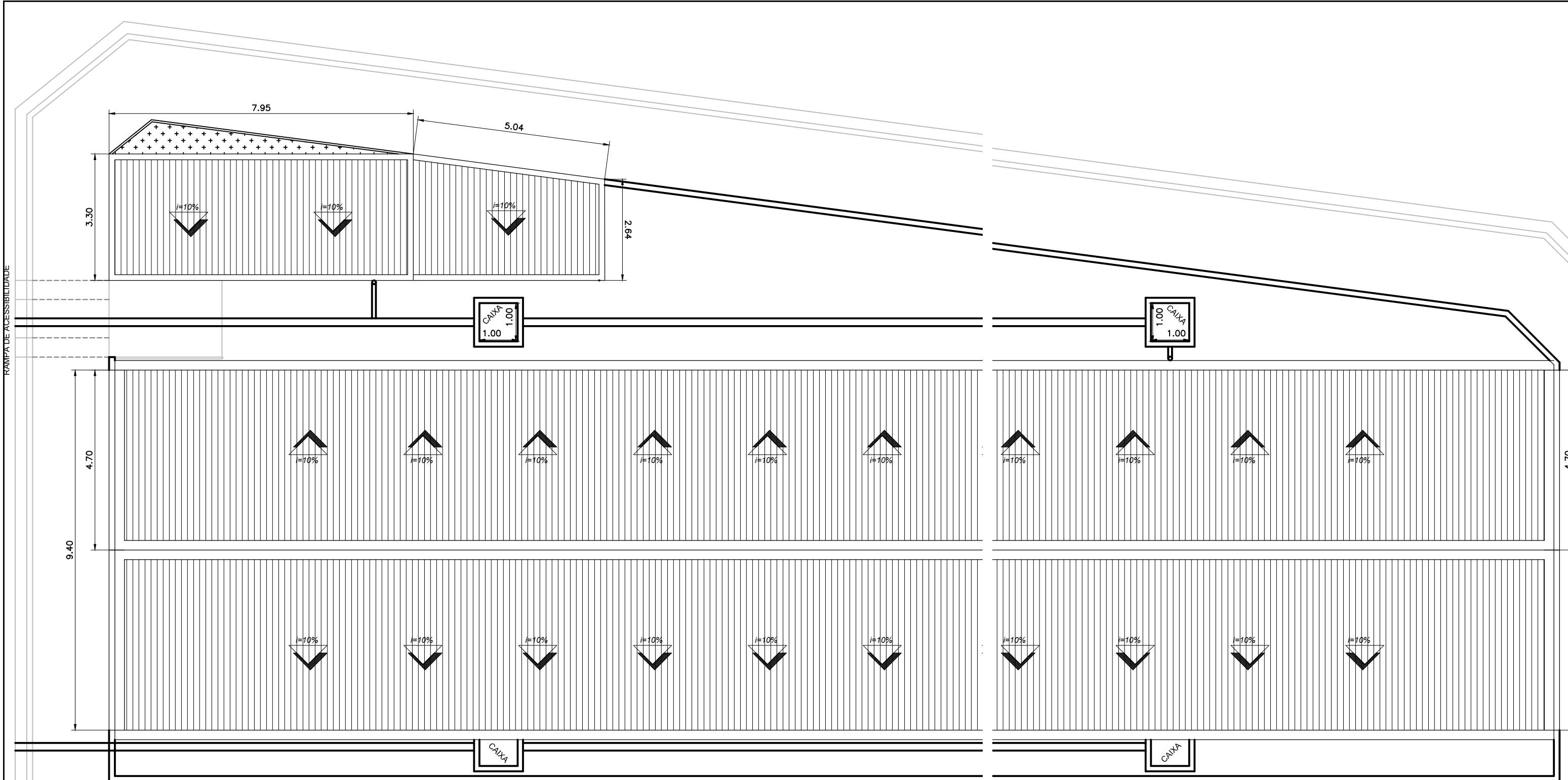
ÁGUA PLUVIAL Escala 1:100
