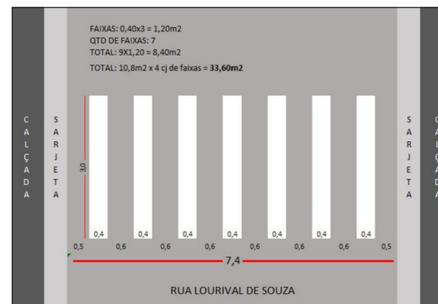
Detalhe Faixa de Pedestre Rua Lourival de Souza
